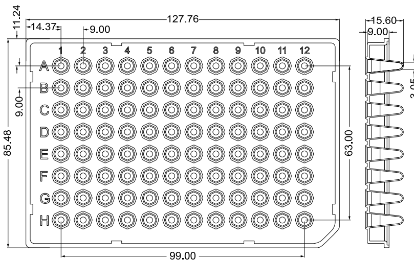
100ul 96 孔 - 半裙边
