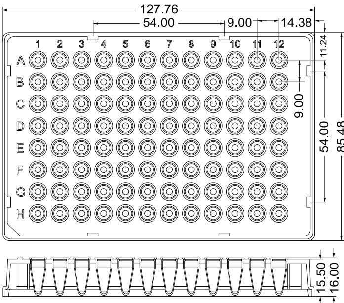
100ul(200ul) 96 孔 - 全裙边 白框，白管
